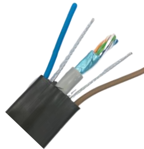
CAT5E + 2c x 0,75 + 2 steel
